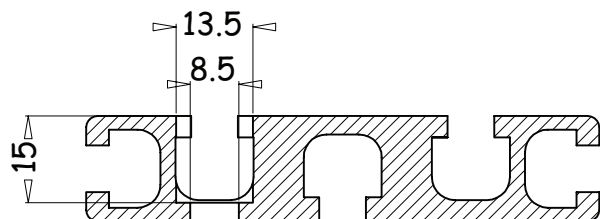
Foratura per TCEIN e TCEIR
