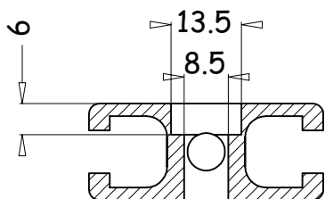
Foratura per TCEIR
