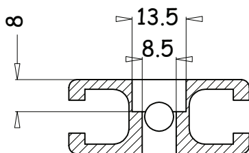
Foratura per TCEIN
