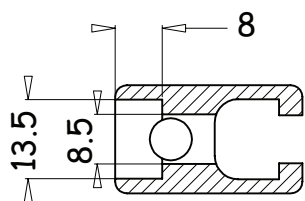
Foratura per TCEIN
