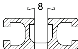
Foratura per TCEIR
