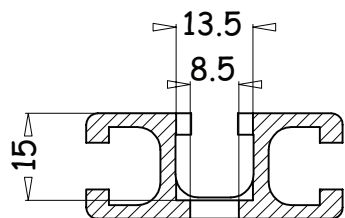
Foratura per TCEIN e TCEIR
