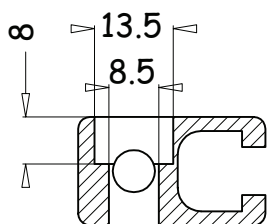
Foratura per TCEIN
