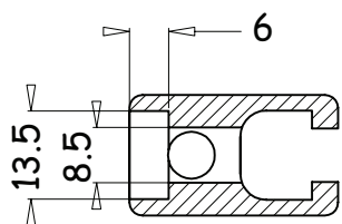
Foratura per TCEIR
