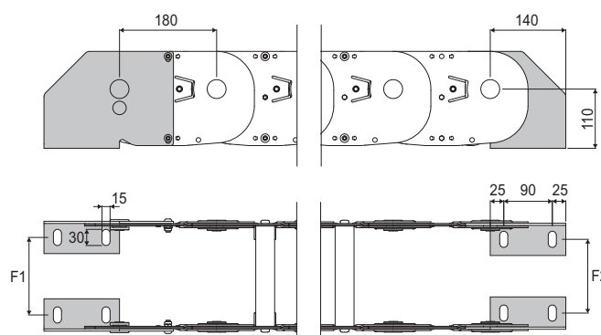
Fig. A Fissaggio della catena sull'esterno raggio. (Fig A) Vedi varianti di montaggio a pag. 31
